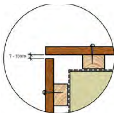
TEKENING B Ventilatie door de horizontale bevestigingsregels op vaste afstanden te onderbreken.
